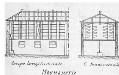
Coupe schématique d'une magnanerie, D. de Prat, Filature - 1ère partie - Fibres animales et minérales, Encyclopédie Roret et Mulo, Paris 1914.
